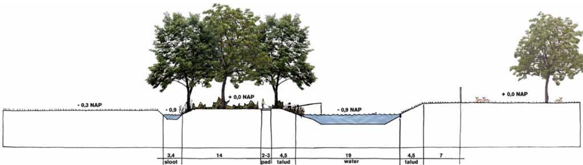
Huidige profiel watergang
