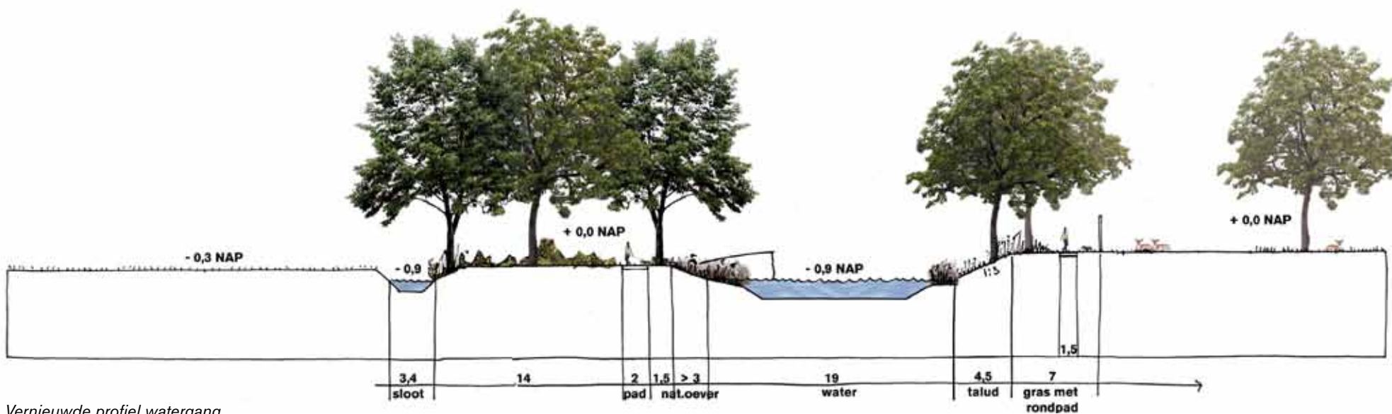
Vernieuwde profiel watergang
